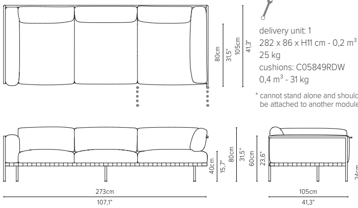
05849RD-x - Right arm corner module 273 cm*
